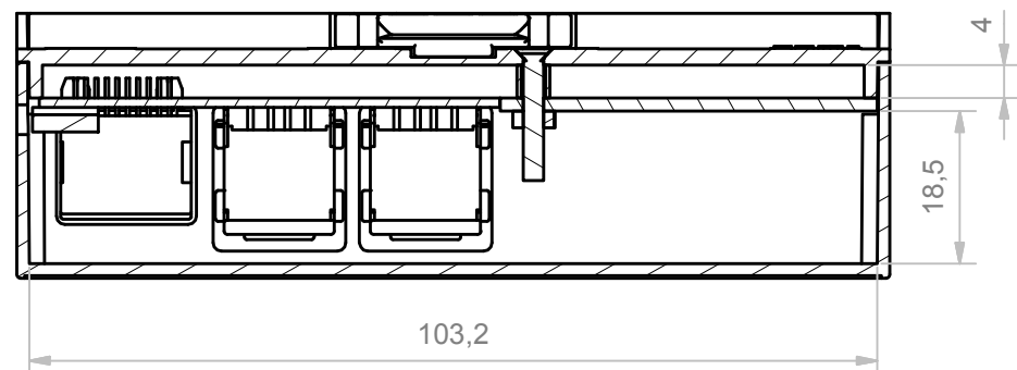
A-A (1:1)
