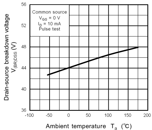
Fig. 9.12 V_{(BR)DSS} - T_a
