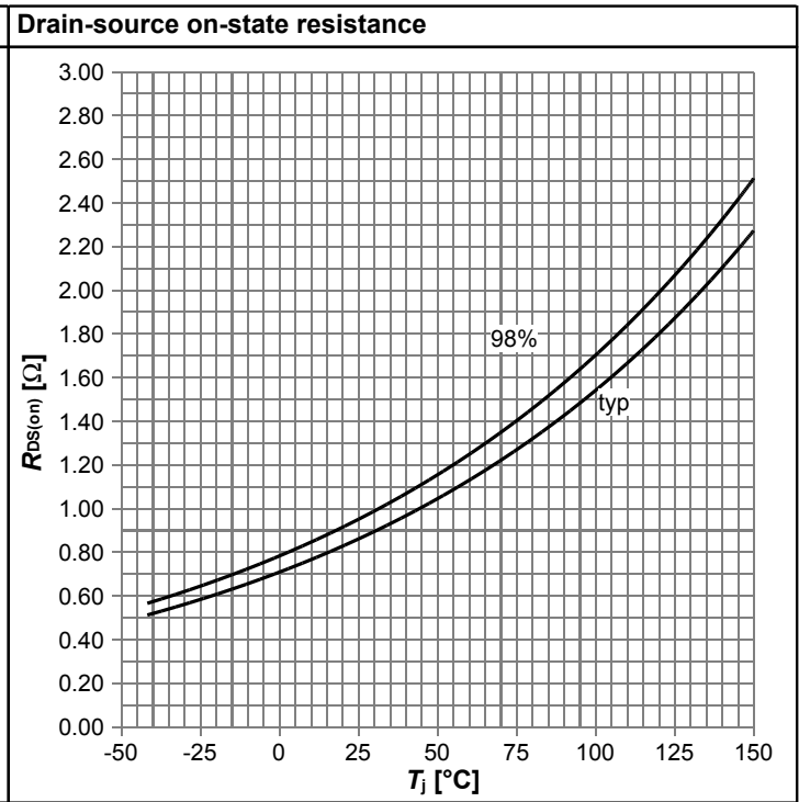
R_{DS(on)}=f(T_j); I_D=1.2\text{ A}; V_{GS}=13\text{ V}
