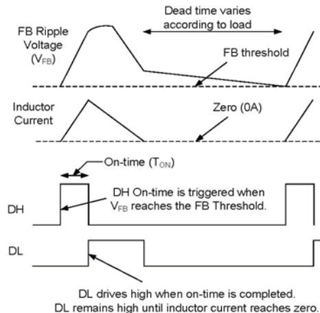
Fig. 6 - Power-Save Mode
