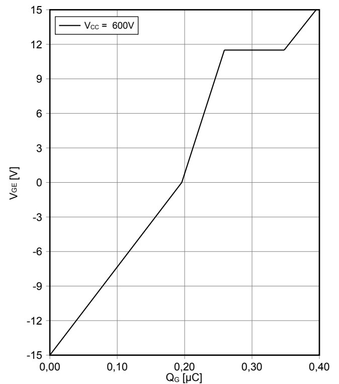
Gateladungs Charakteristik IGBT, Wechselrichter (typisch) gate charge characteristic IGBT, Inverter (typical) V_{GE} = f(Q_G) I_C = 25\text{ A} , T_{vj} = 25^\circ\text{C}
