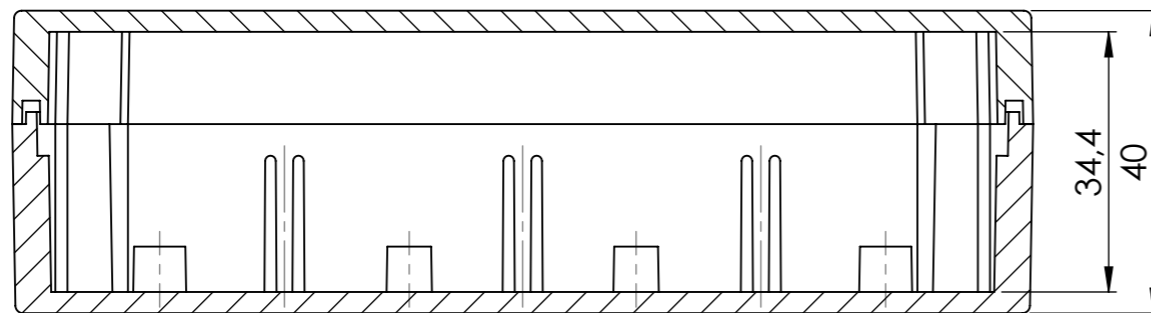
SECTION A-A
