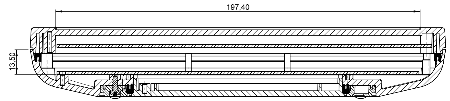
Gehäuseunterteil Innenansicht Bottom part of case inside view
