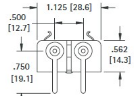
CAT. NO. 303-P PC Lugs
