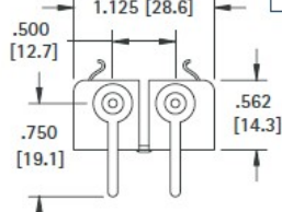
CAT. NO. 1291-79 PC Lugs
