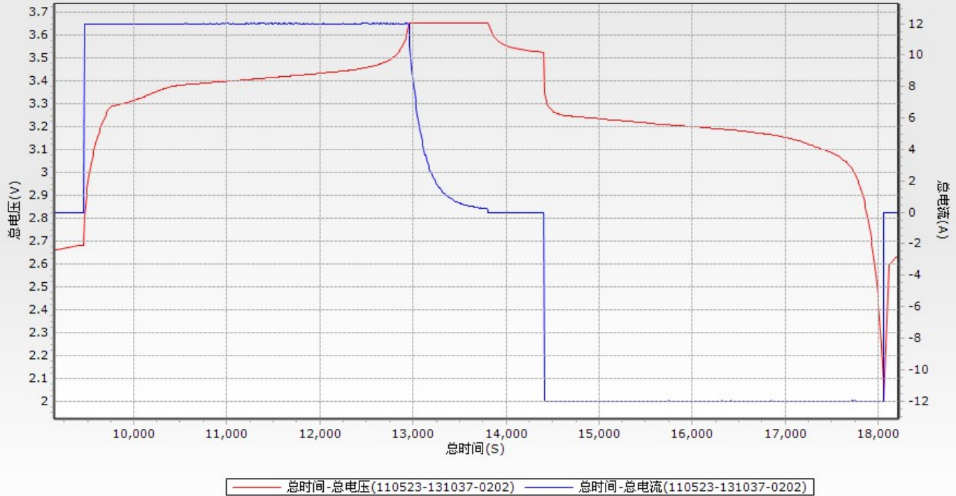
38140S (12Ah) 1C充放曲线图
