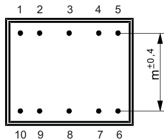
KK 42/EI 08-4
