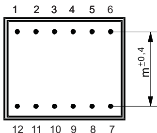
KK 42/EI 07-4
