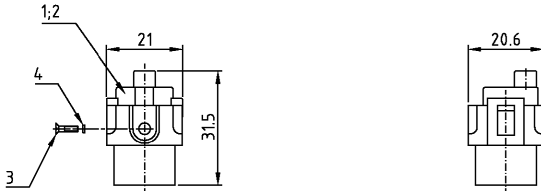
Maßbild Outline drawing
