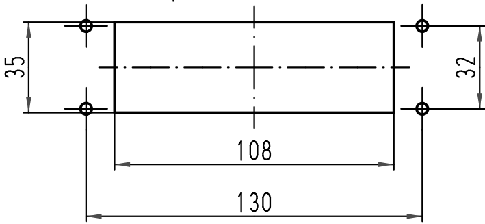
1:2 Montageausschnitt panel cut out
