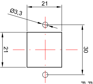
Panel cut out Foratura del pannello
