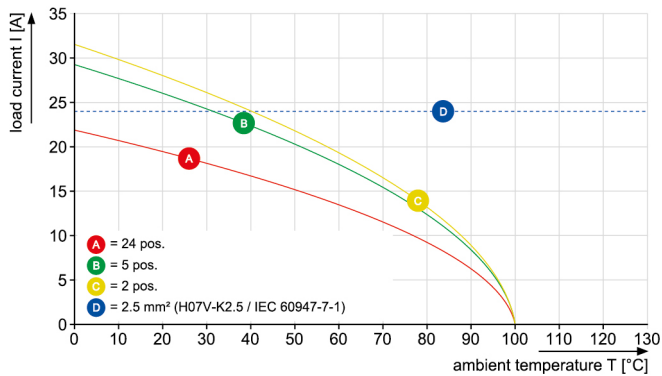
BLT 5.00HC/././180 - SL-SMT 5.00HC/././90
