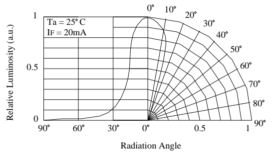
Directivity (Angle : 30°)
