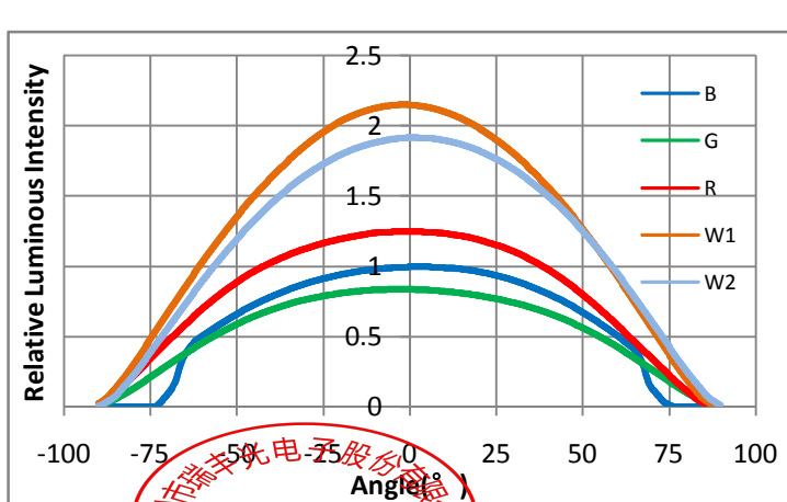
Fig.6-Radiation diagram 辐射特性曲线
