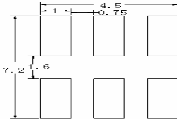
建议焊盘尺寸
