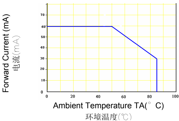
Forward Current Derating Curve 环境温度与电流的关系曲线图
