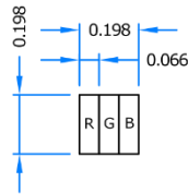
DETAIL A 60:1
